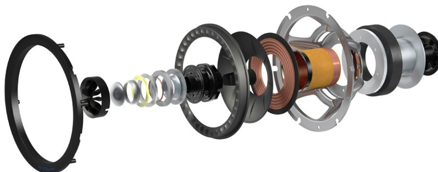
Die Detailgrafik veranschaulicht den komplexen Aufbau des koaxialen Uni-Q-Töners
