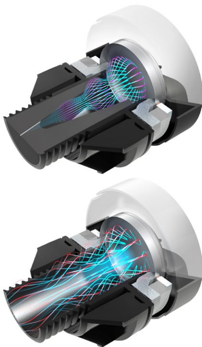
Durch die Bedämpfung des rückwärtigen Kammervolumens wird die Hochtonwiedergabe verbessert. Das Bild oben zeigt die Schallausbreitung mit Bedämpfung, das Bild unten ohne
